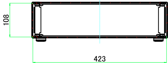
A-A (1:7)
